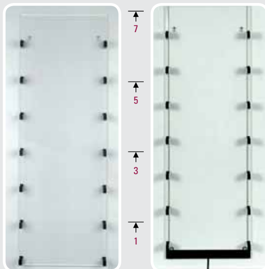
Wandhalterungen (WH) gibt es mit und ohne Stromzuführung in verschiedenen Größen von 1–7 Auflagermöglichkeiten.
