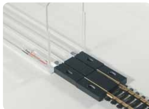
Das Gleisübergangsstück (GU) kann auch in Kombination mit einem Gleisadapter (GA) verwendet werden, wodurch Röhren mit Spurrillen und Röhren mit Metall-Schienen flexibel am selben Anschlussgleis eingesetzt werden können.
